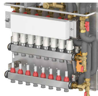
Příklad podlahového rozdělovače se svorkovnicí (obr. podobný)
