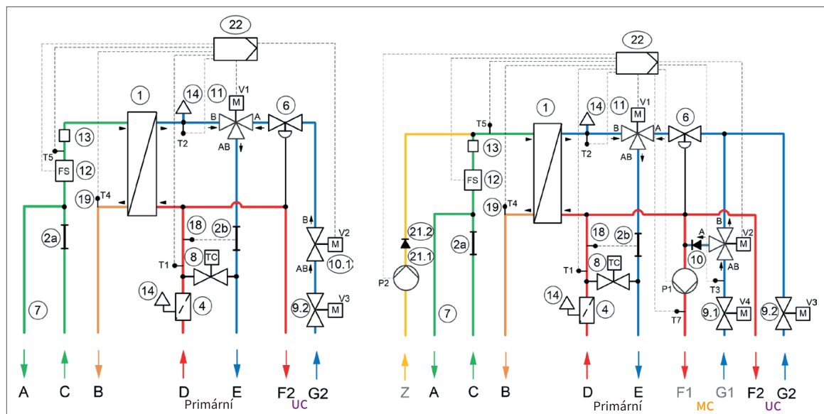
LogoMatic G2 MC-UC DHWC (příkl. s volitelnou CPV)
